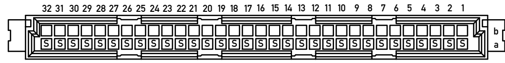
Bestückungsplan / contact layout
