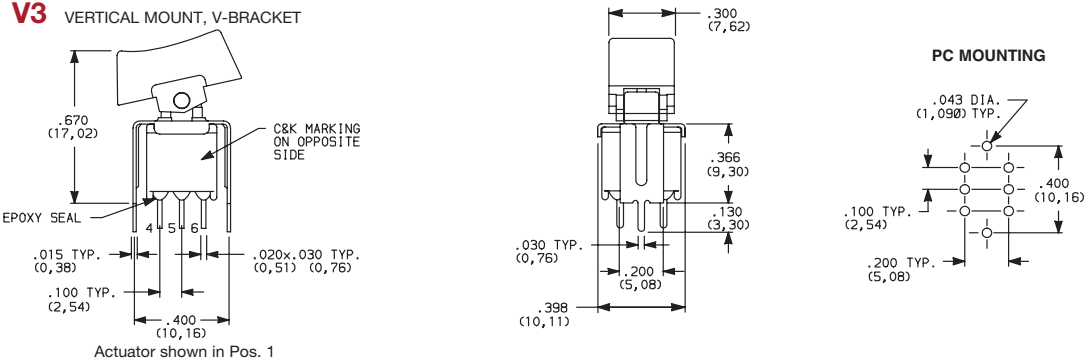
ET21J1V3BE2 DPDT
