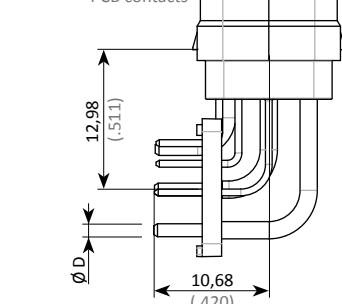
Module à picots soudés Module with angled PCB contacts
