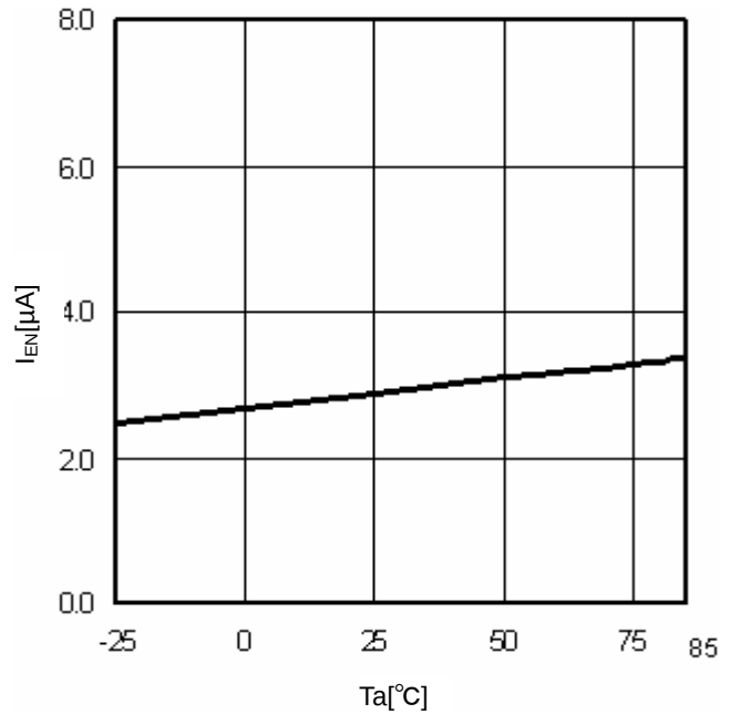
Fig.11 T_a - I_{EN}
