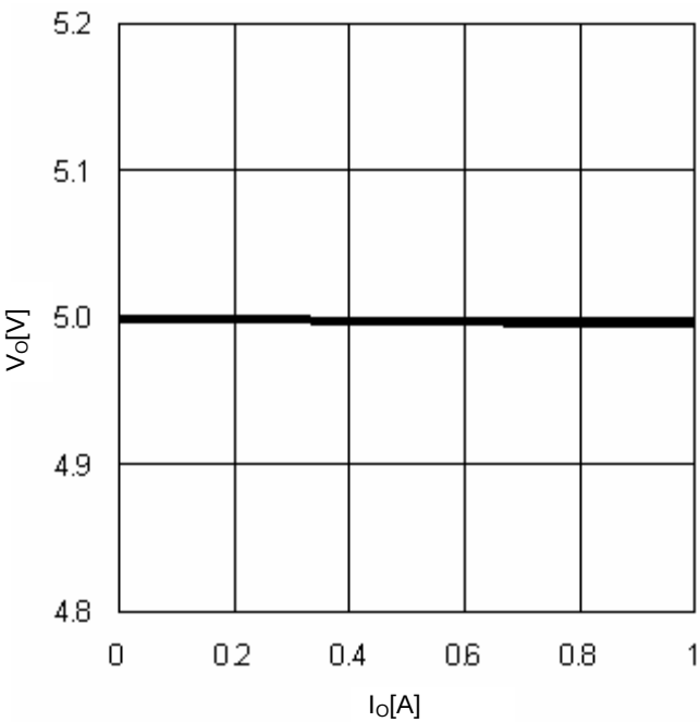
Fig.12 I_O - V_O
