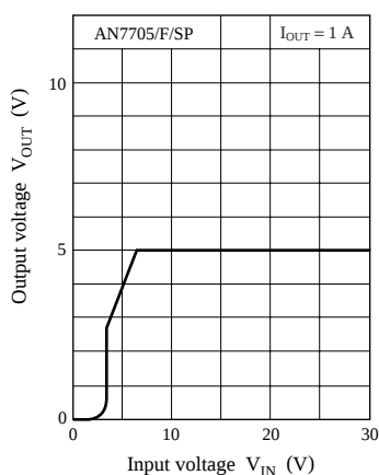
V_{OUT} - V_{IN}
