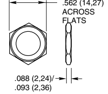
Hex Nut
