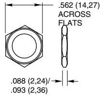
Hex Nut
