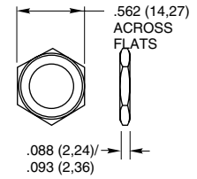
Hex Nut
