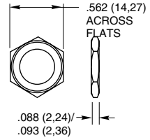
Hex Nut
