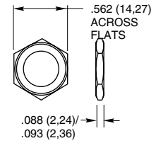
Hex Nut
