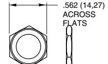
Hex Nut
