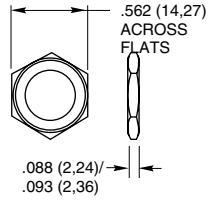
Hex Nut
