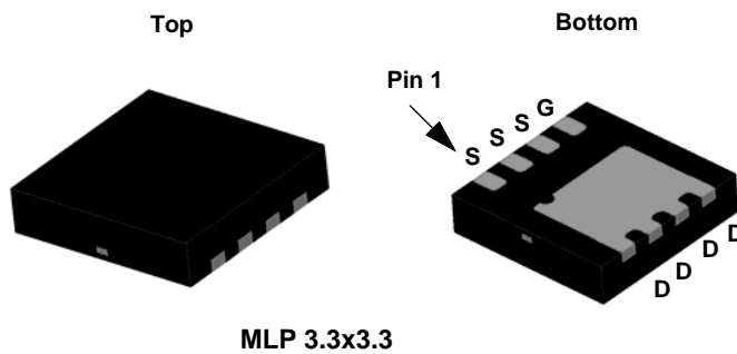
MLP 3.3x3.3
