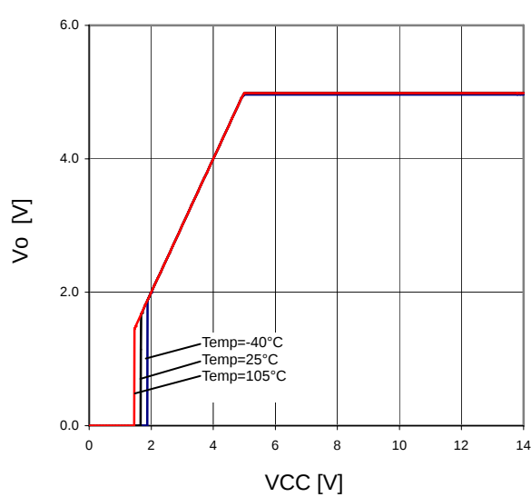
Figure 27. Vcc-Vo (Io=0mA)
