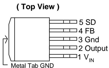
TO263-5L
