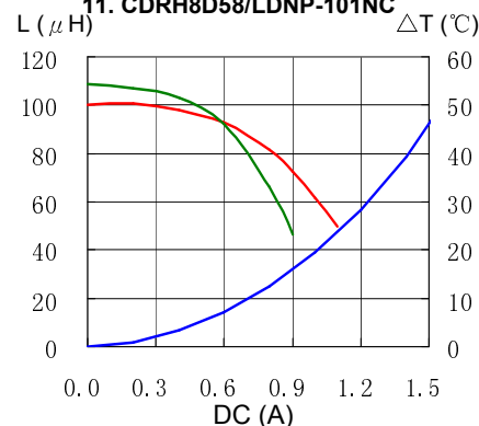
11. CDRH8D58/LDNP-101NC
