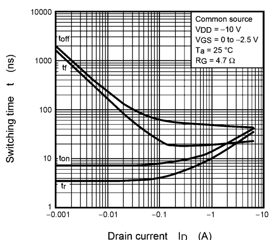
Fig. 7.10 t - I_D
