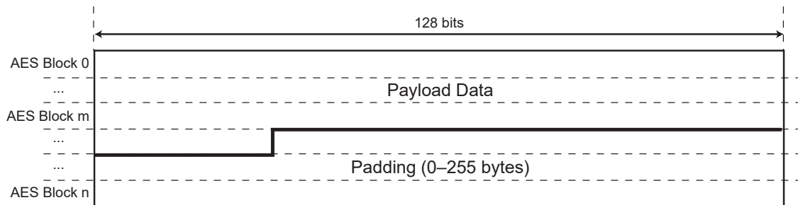
Figure 59-10. SSL Padding
