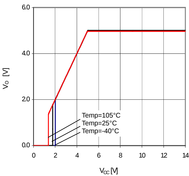
Figure 27. V_{CC}-V_O ( I_O=0\text{mA} )
