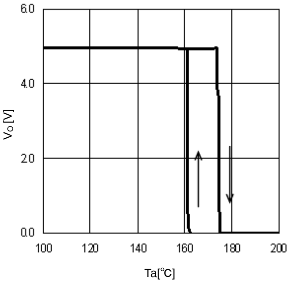
Figure 28. TSD ( I_O=0\text{mA} )
