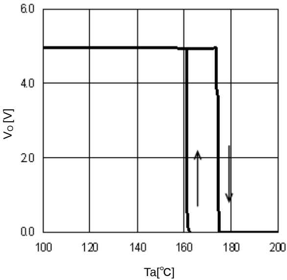
Figure 28. TSD ( I_O=0\text{mA} )
