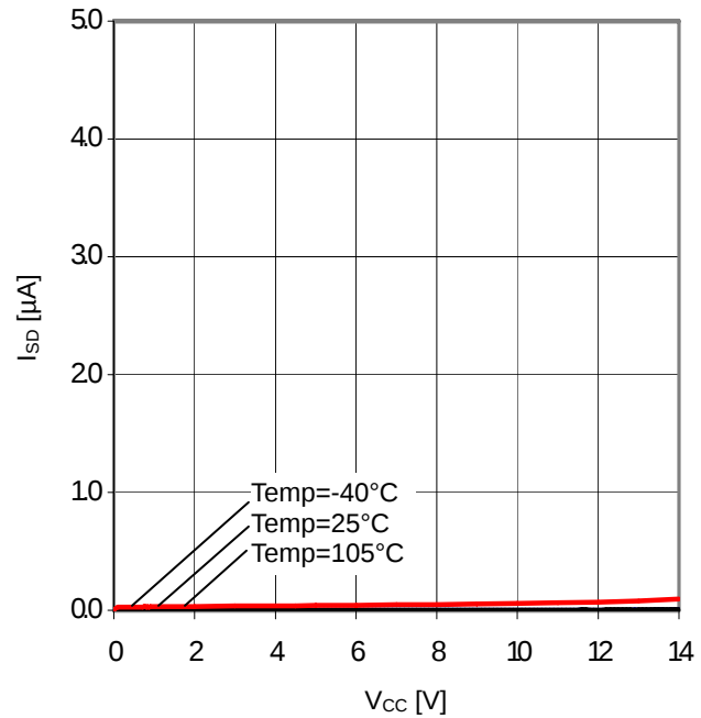
Figure 26. V CC -I SD (V EN =0V)
