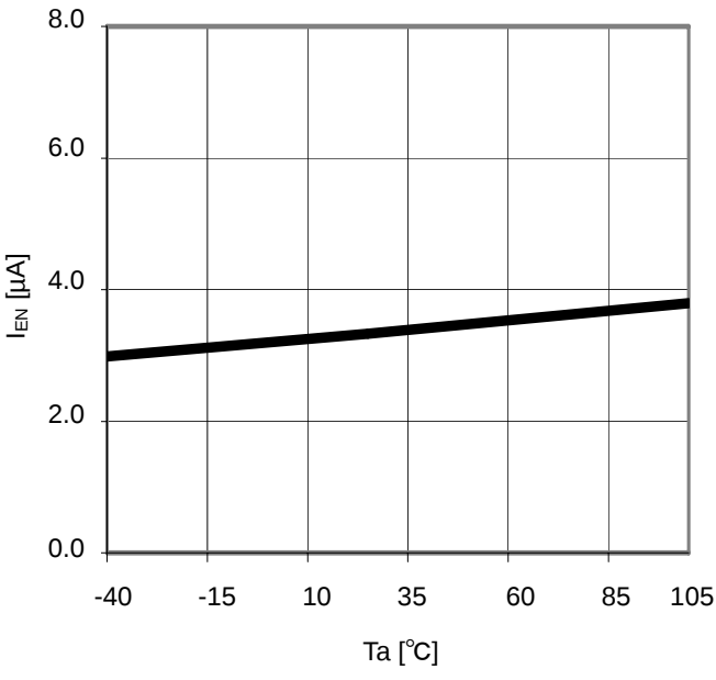
Figure 24. Ta-I EN
