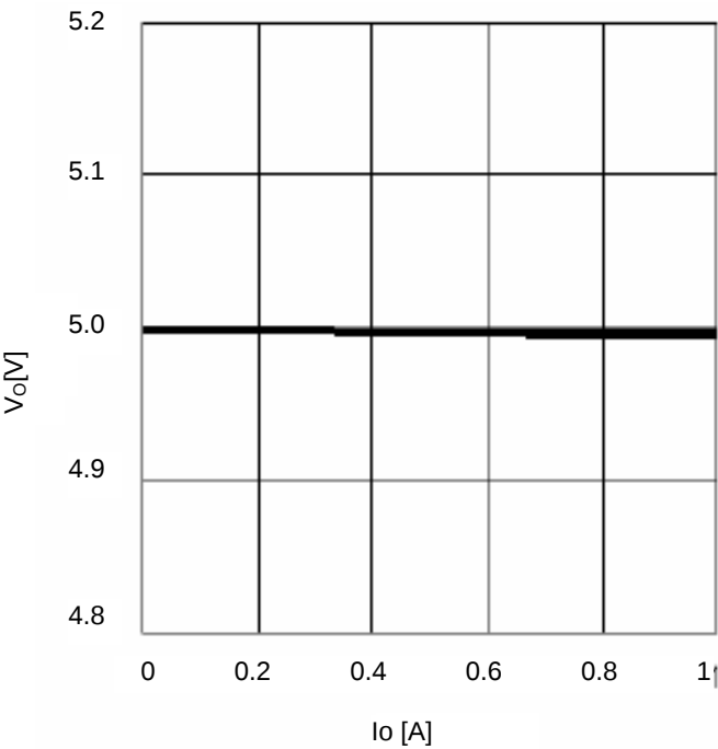
Figure 25. I O -V O
