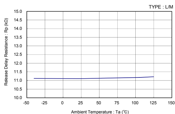
XC6133
