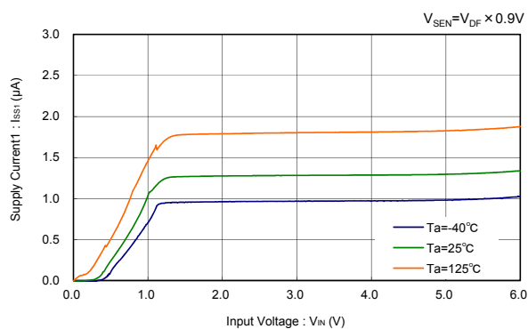
XC6133
