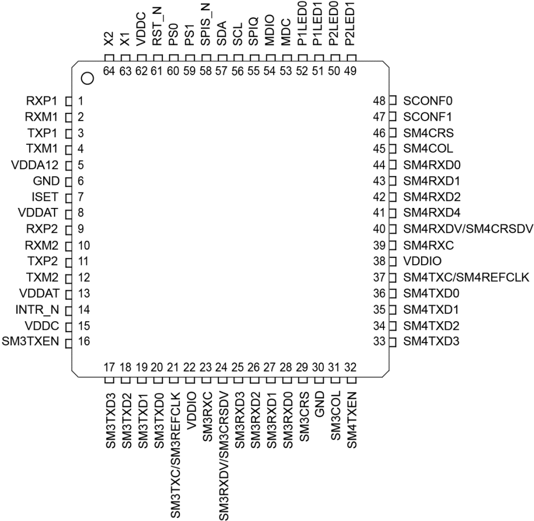
64-Pin QFN
