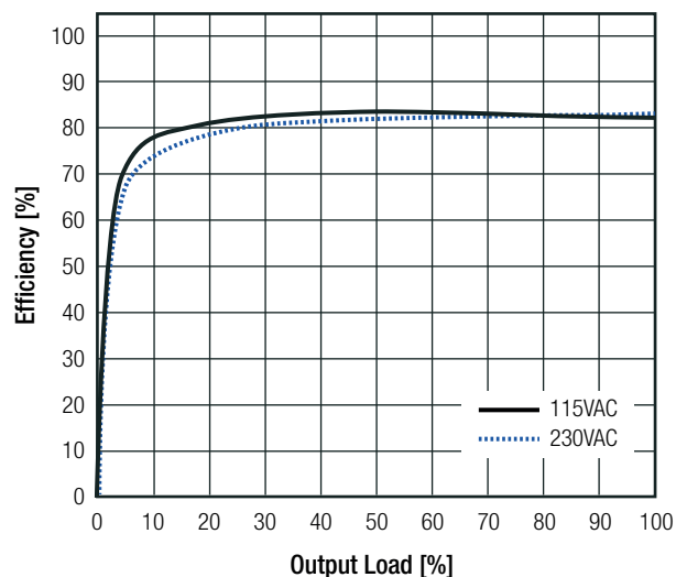
RAC05-15SK
