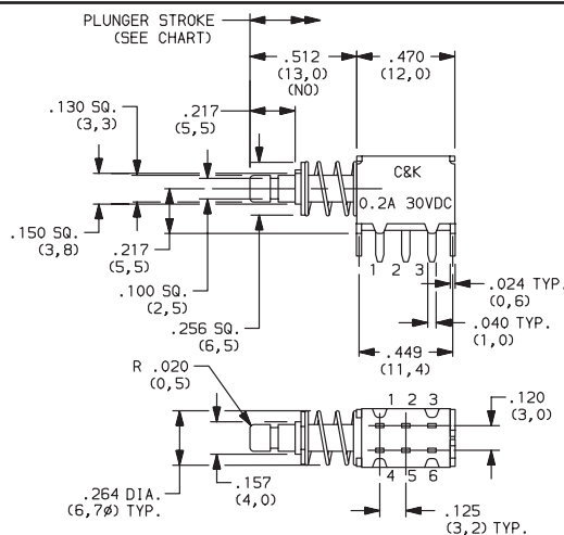
PN21LASA03QE DPDT
