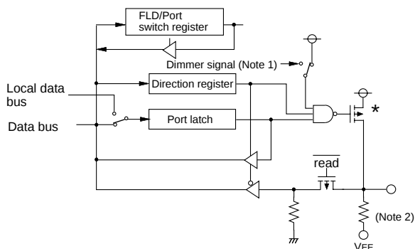
(3) Port P20
