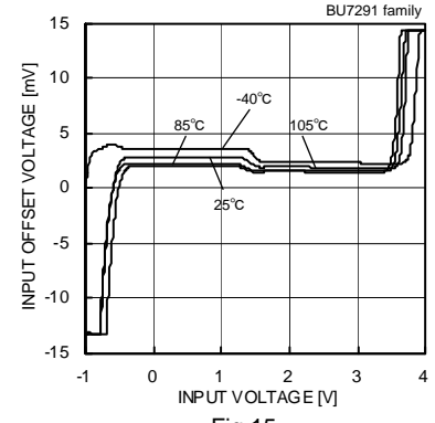
Fig. 15 Input Offset Voltage – Input Voltage (V DD =3[V])
