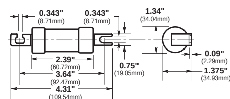
CGL 70-100
