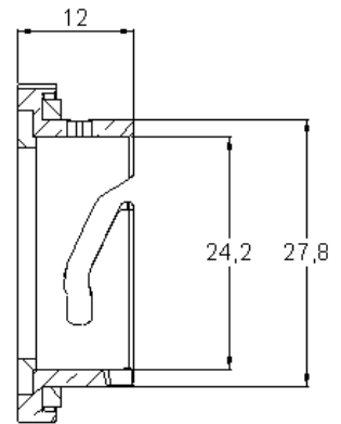
COUPE A-A
