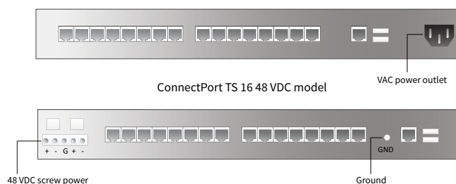
ConnectPort TS 16 (EIA-232 and MEI AC models)
