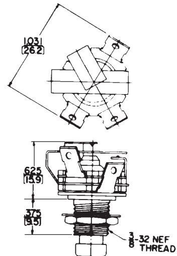
SPDT 1-C
