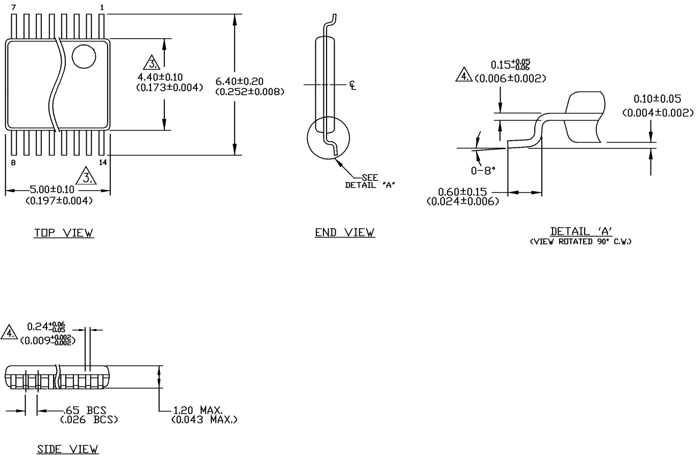
14-Pin TSSOP (TS)
