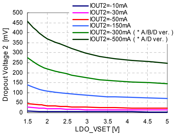
RP600Kxxxx, Ta=25°C
