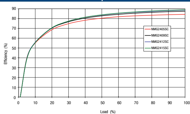
24V Input
