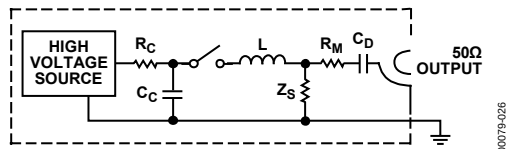
Figure 26. EFT Generator
