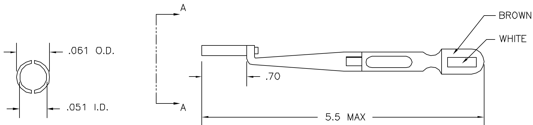
VIEW A-A
