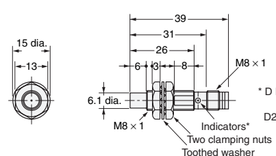
Diagram 29 E2E-X4MD□-M3G/E2E-X2ME□-M3/X2MF□-M3
