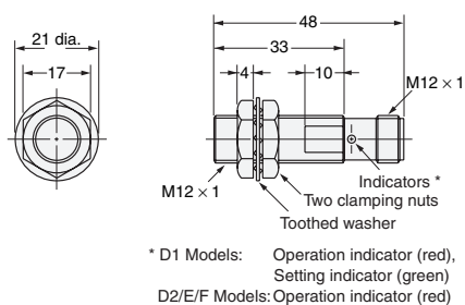
Diagram 22 E2E-X2Y□-M1
