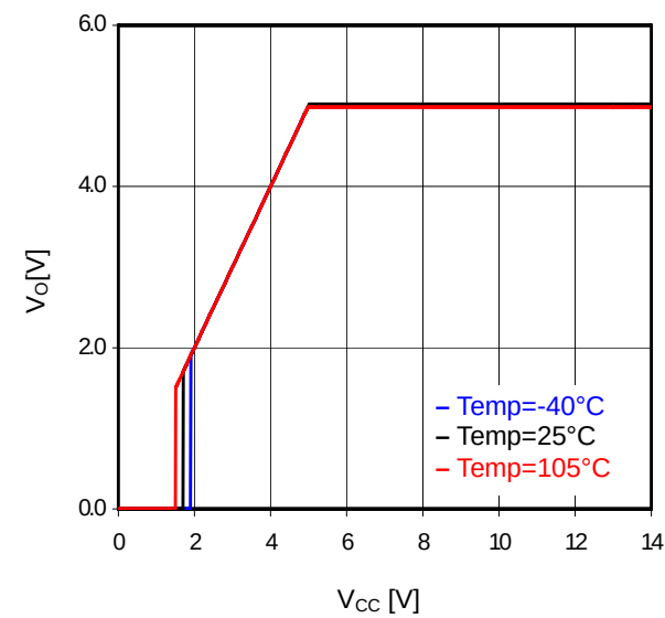
Fig. 27 V_{CC}-V_o ( I_o=0mA )
