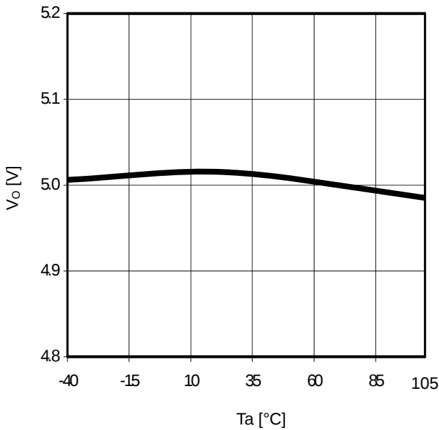
Fig. 21 Ta-V_O ( I_O=0mA )
