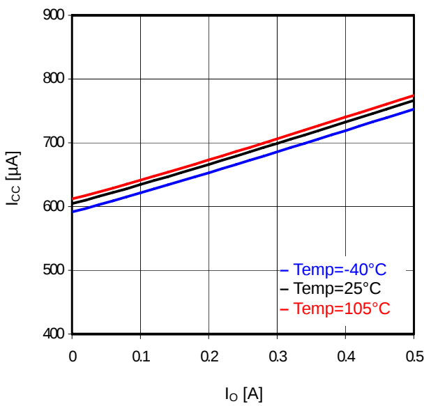
Fig. 30 I_O-I_{CC}
