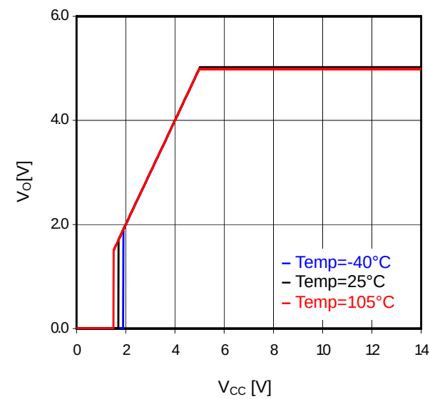
Fig. 27 V_{CC}-V_O ( I_O=0\text{mA} )
