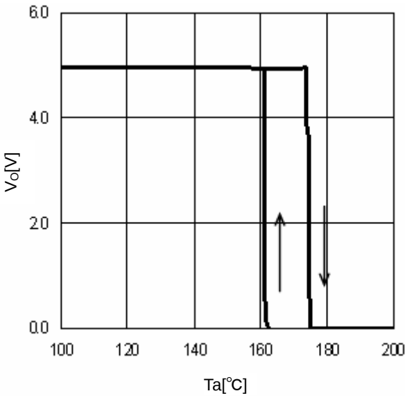
Fig. 28 TSD ( I_O=0mA )
