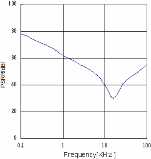
Fig. 32 PSRR ( I_o=0mA )
