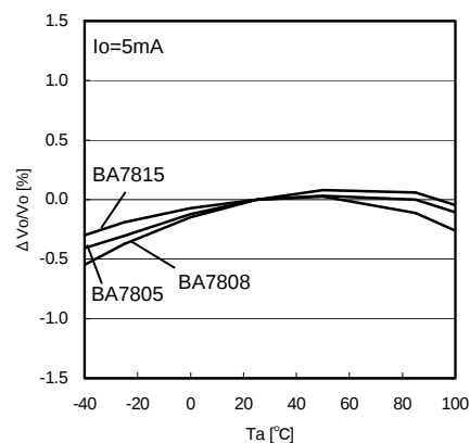
Fig.22 T_a - V_o
