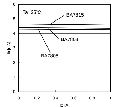
Fig.24 I_o - I_b
