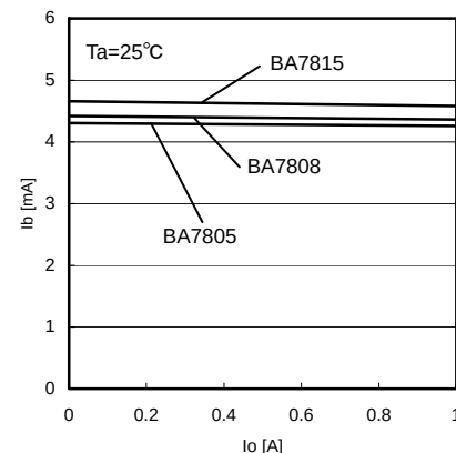
Fig.24 I_o - I_b
