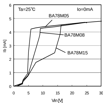
Fig.4 V_{in} - I_b
