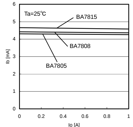
Fig.24 I_o - I_b
