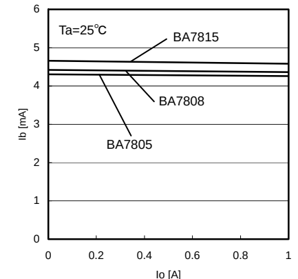
Fig.24 I_o - I_b
