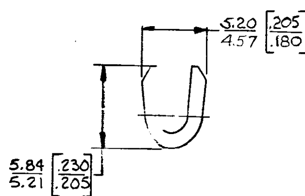
SEC A-A
