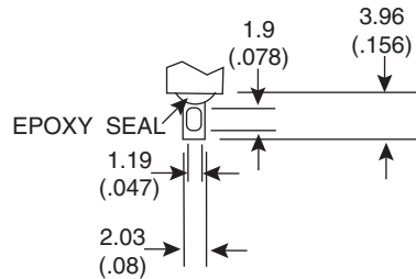
SOLDER LUG
