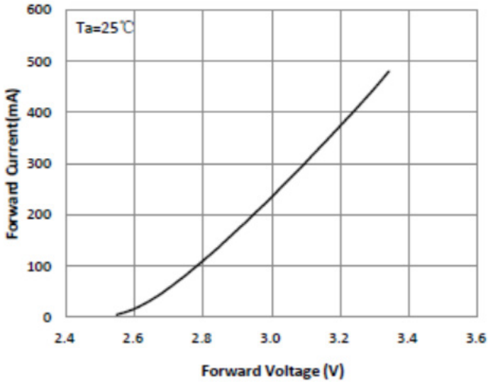
V_f ----- I_f
